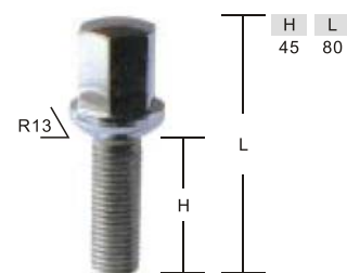
WB007 17mm HEX Ø23mm
